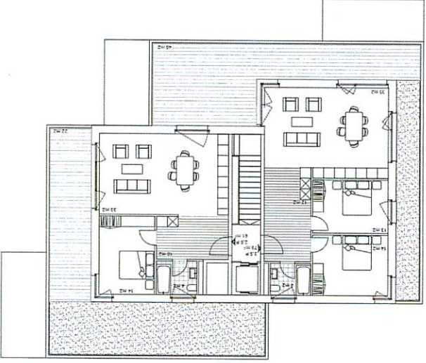
Attique 1/100
