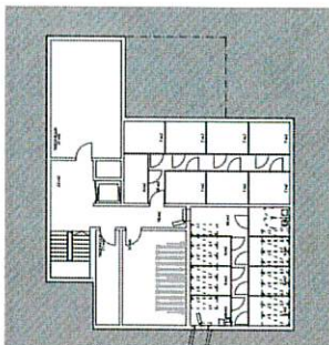
Sous-sol-2 1:200
