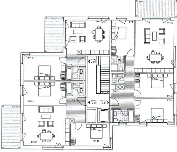
Etage type 1/100
